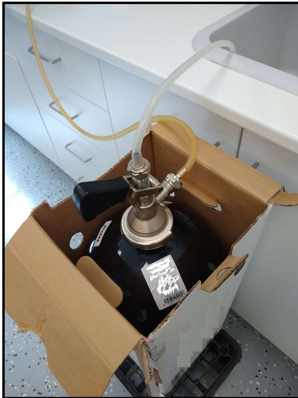
Obr. 17 Následné čepování vody z obalu PETAINER KEG
